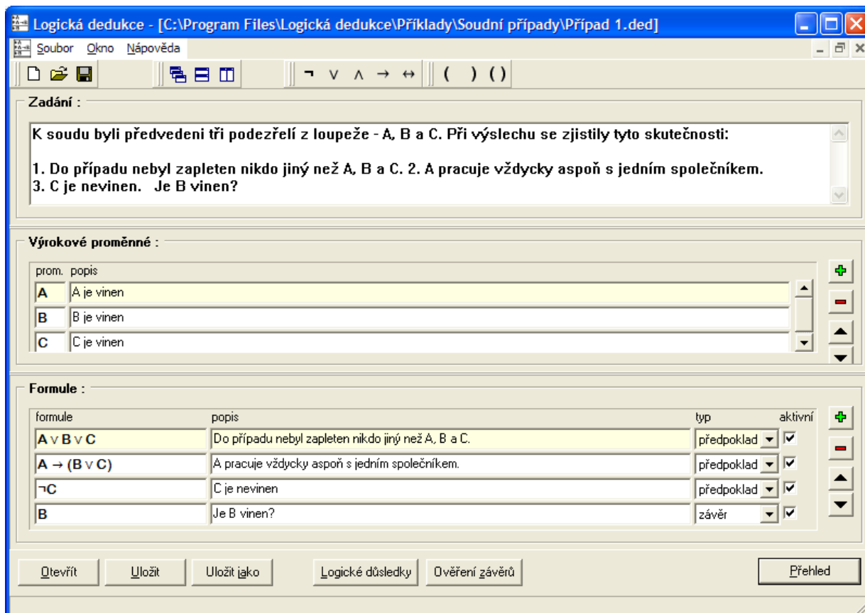
Obrázek 1: Grafické rozhraní aplikace pro dedukci
